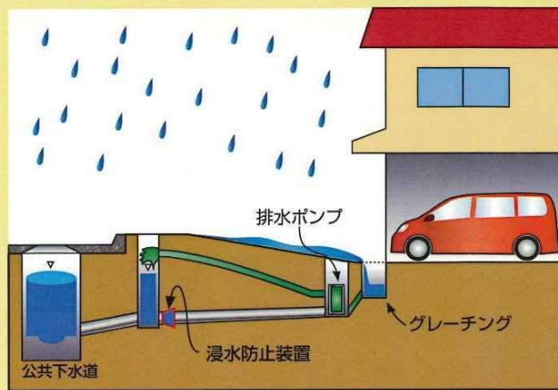
B 自然流下排水(通常排水)+ポンプ排水(浸水時)+逆止弁・仕切弁等
