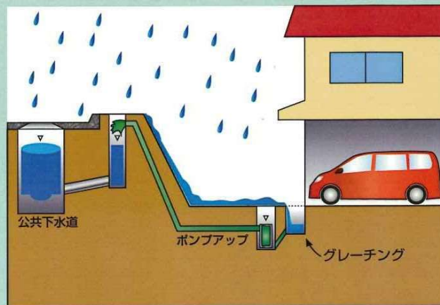
D ポンプ排水(常時排水)
