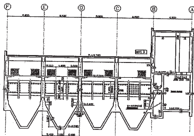
⑩~⑦ 断面图
