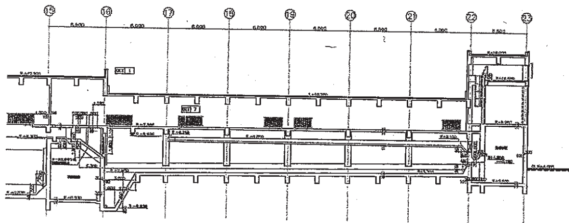
⑤~④ 断面图
