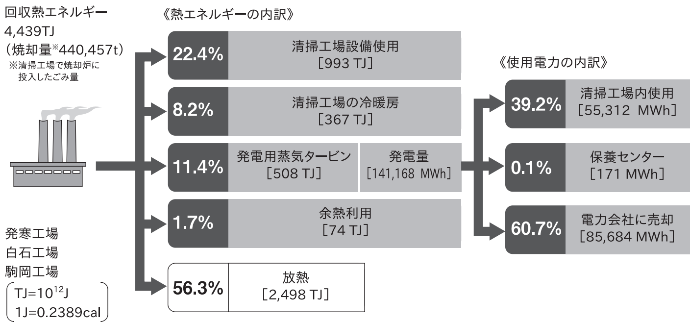
図2-3-15 清掃工場の熱利用(2023年度実績)
