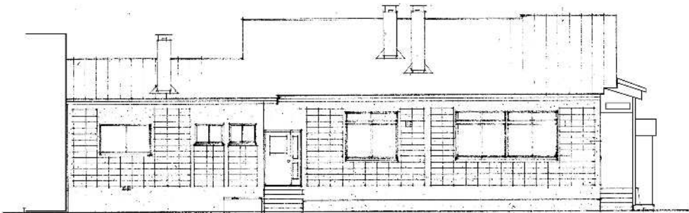
西立面图
