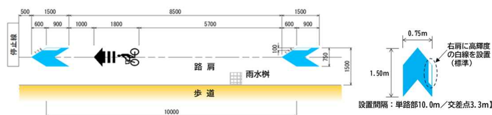
図 矢羽根型路面表示の標準整備図
