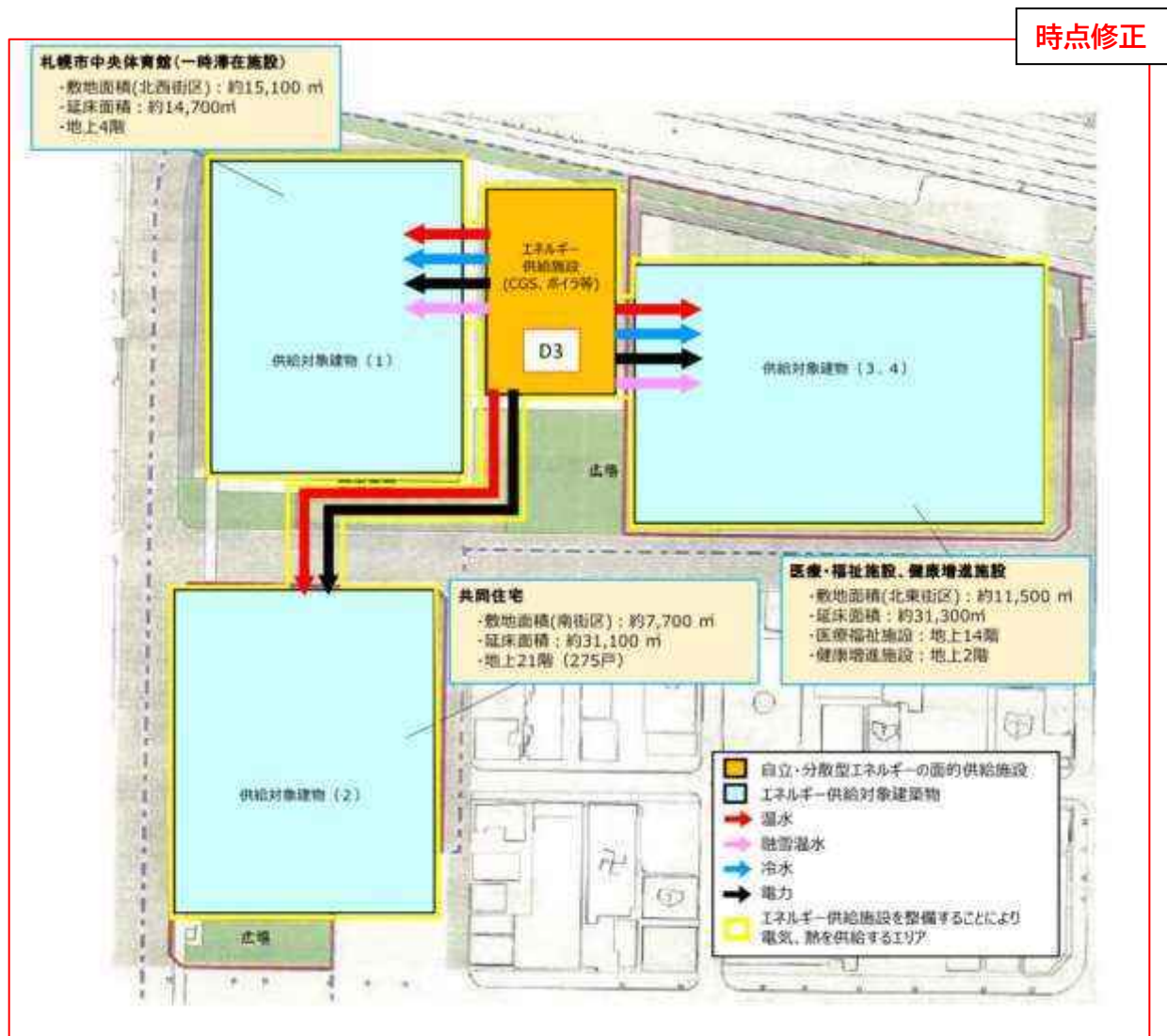
図 17 札幌駅・大通駅周辺地区都市再生安全確保計画図 D3 4 6 エネルギーセンター詳細
