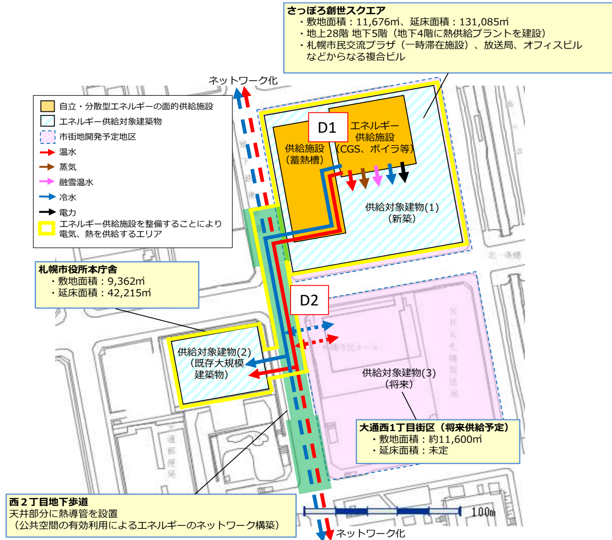
図 16 札幌駅・大通駅周辺地区都市再生安全確保計画図 D1 創世エネルギーセンター及び D2 西2丁目地下歩道熱導管ネットワーク 詳細
