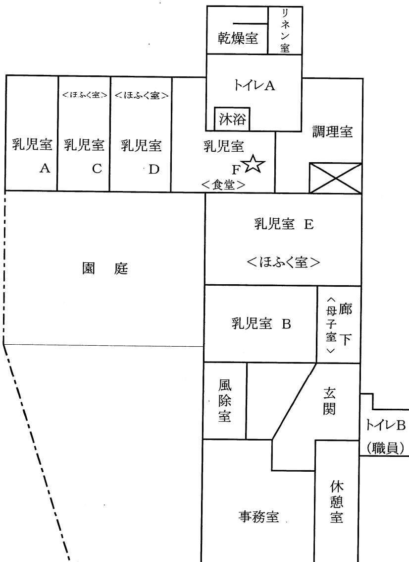
建物の略図
