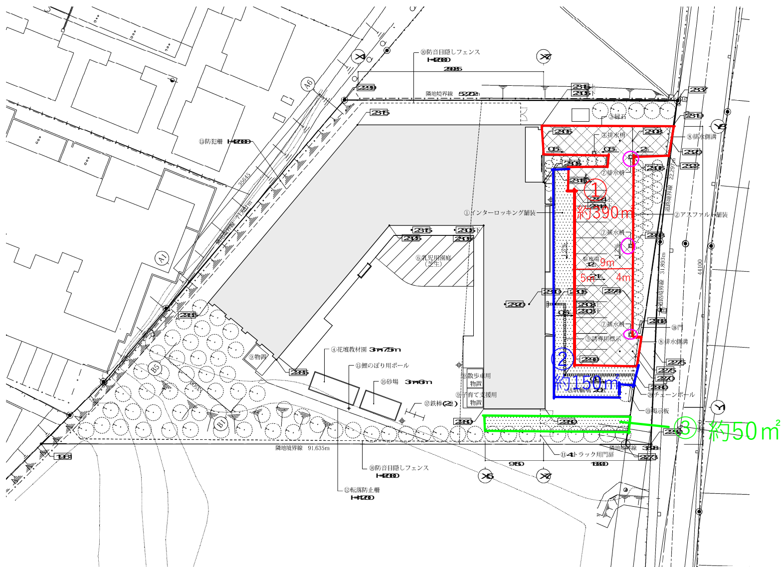
厚別区保育・子育て支援センター外溝図
