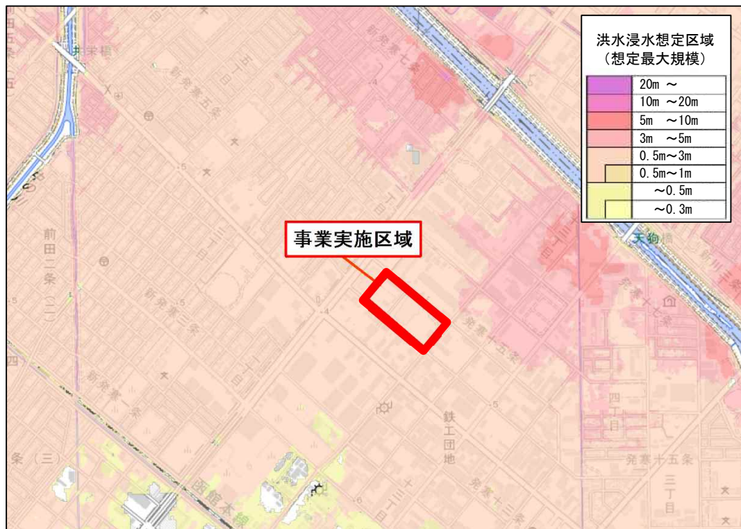
図 6.6 新発寒清掃工場周辺の想定最大規模時（1,000 年に 1 度）の浸水深さ
