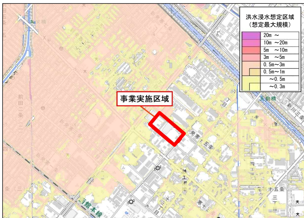
図 6.5 新発寒清掃工場地周辺の計画降雨時（100 年に 1 度）の浸水深さ
