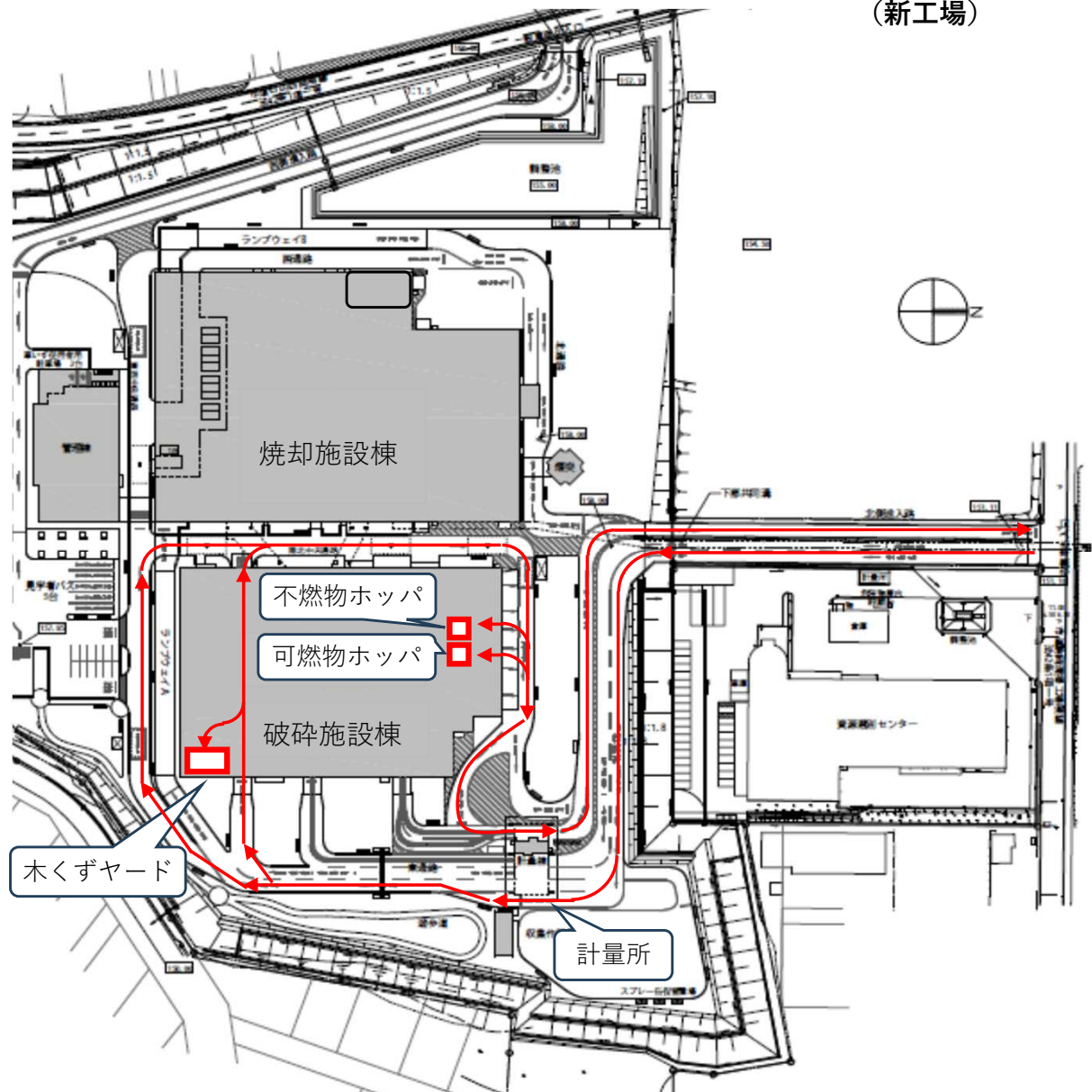
駒岡清掃工場破碎処理物等運搬業務 構内平面図
