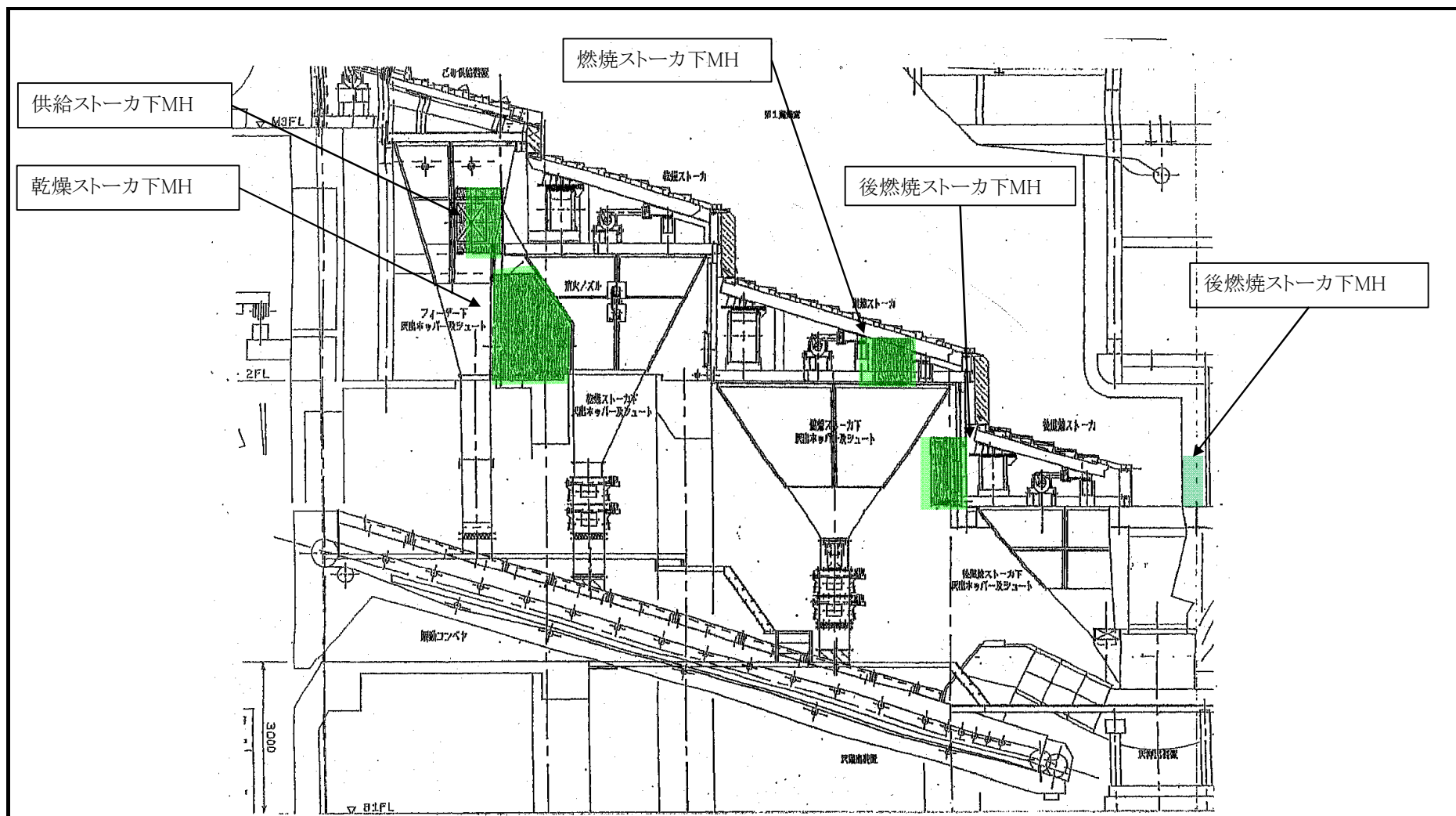
ストーカ下養生範囲図
