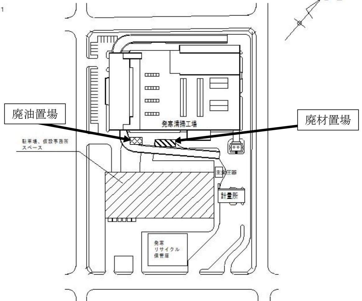
発寒清掃工場配置図 1:2000
