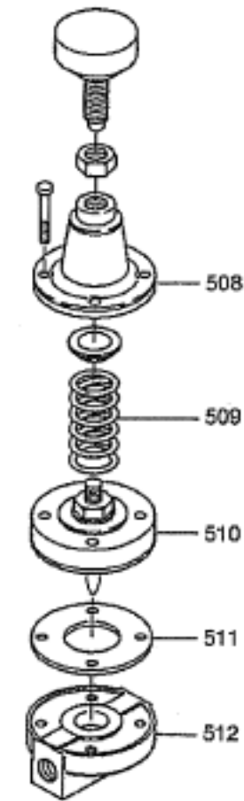
圧力調整弁 507
