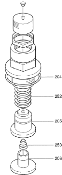
調圧逆止弁 203
