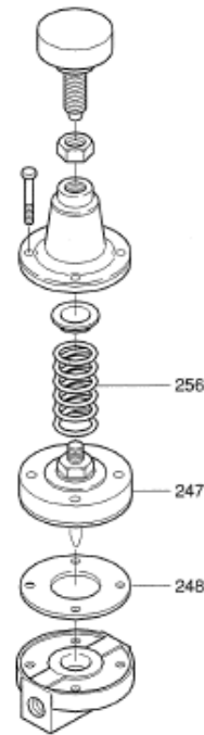
圧力調整弁 246
