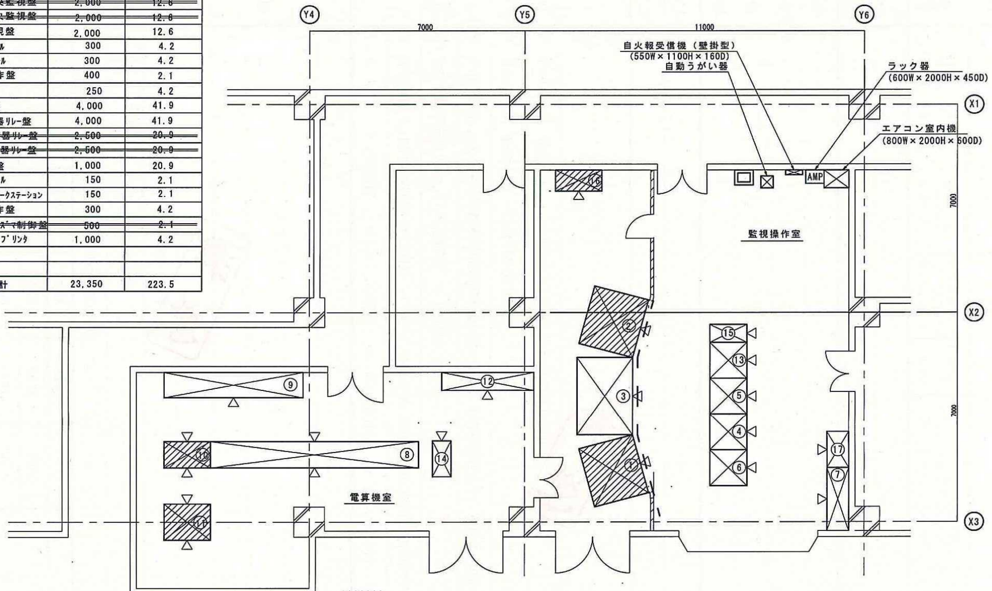
4階 監視操作室・電算機室配置図
