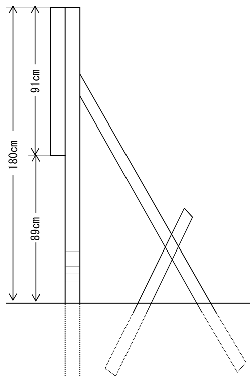
（側面図・全区画共通）
