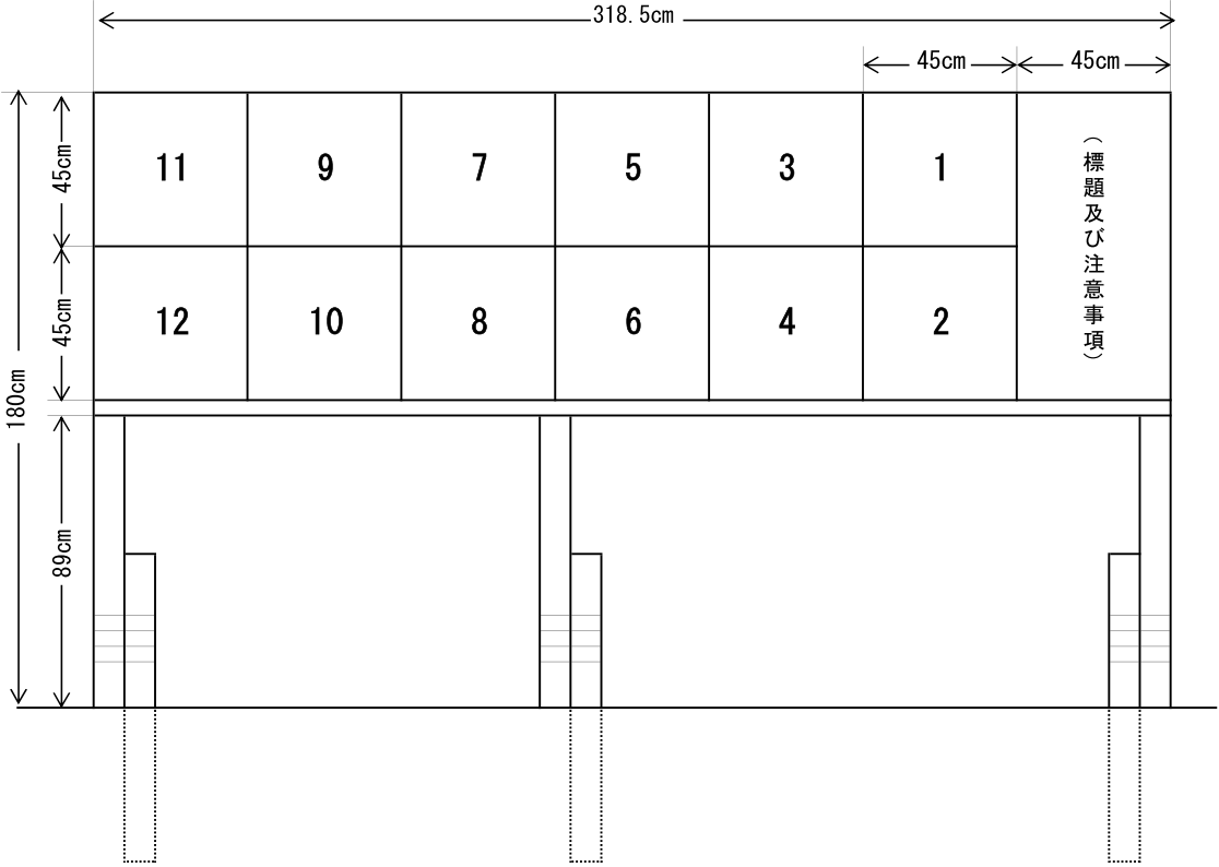
(背面図)
