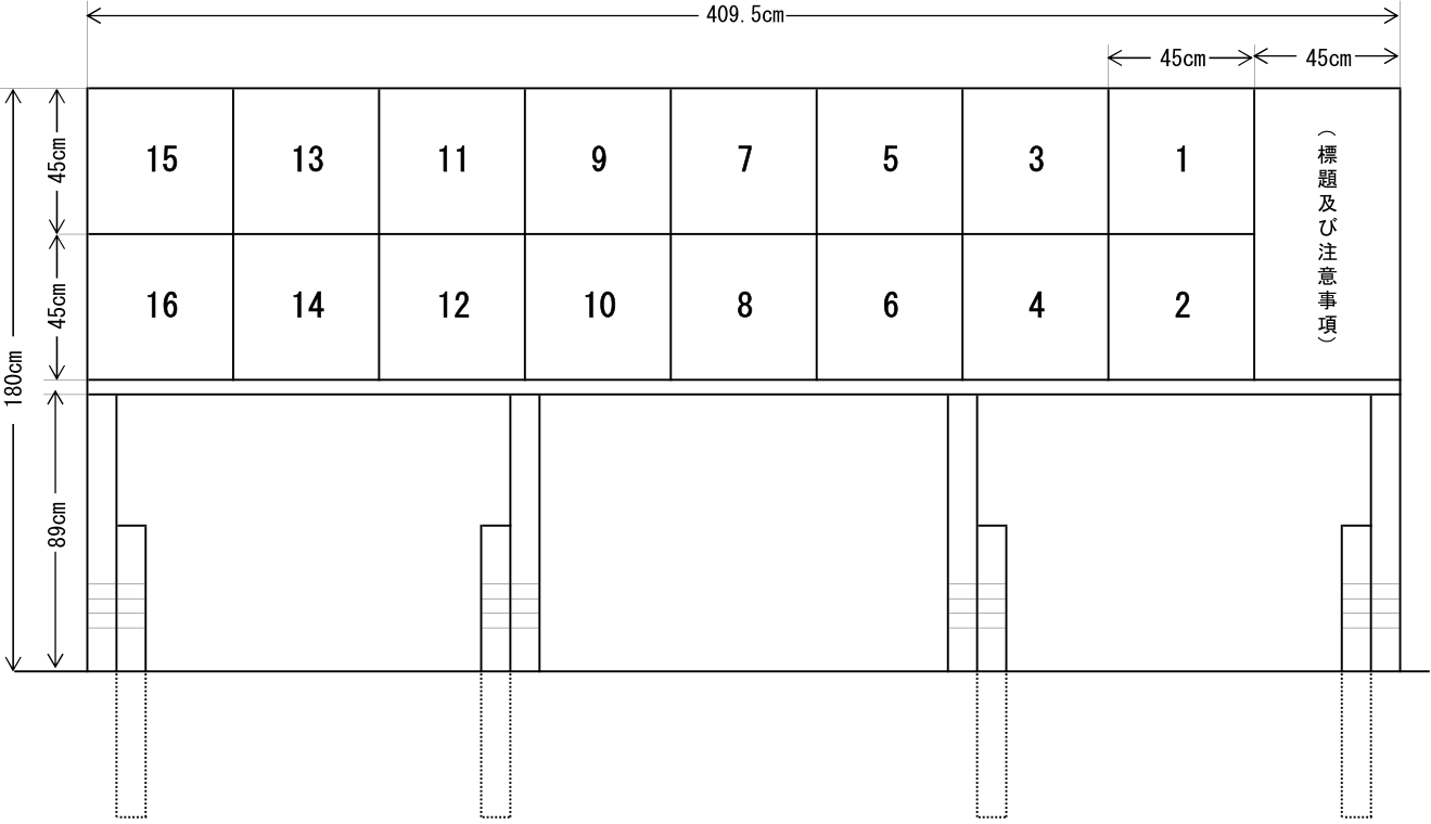
(背面図)
