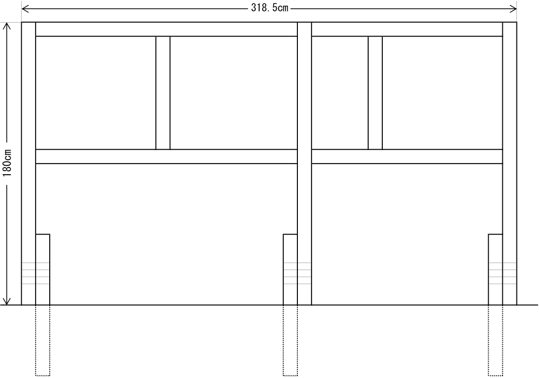
(背面図)
