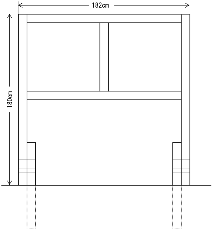
(背面図)
