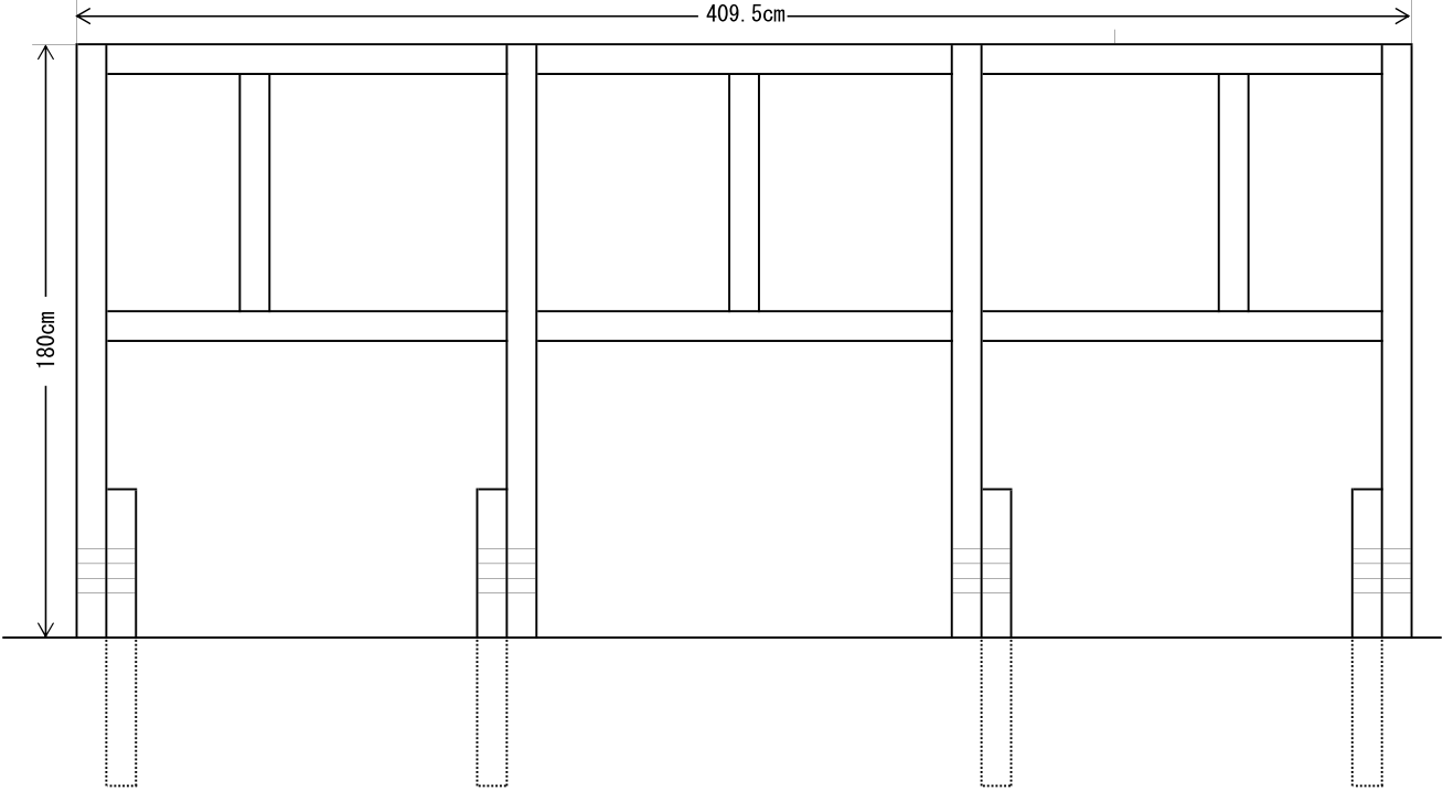
(背面図)
