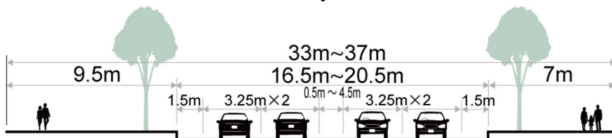
図2 幅員構成
