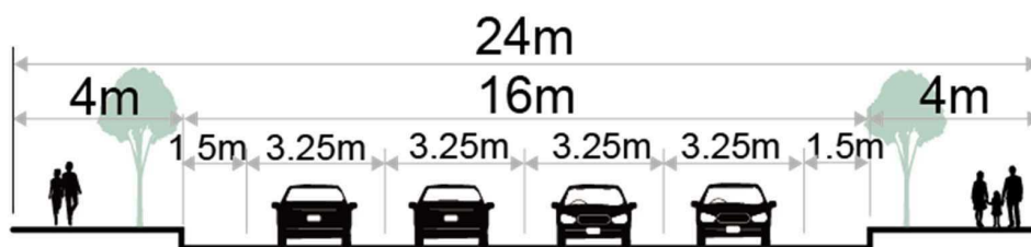
図1 幅員構成
