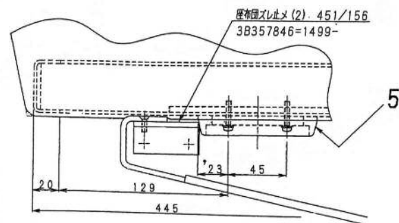
A部詳細
