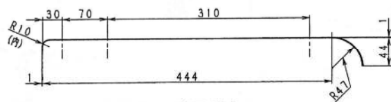
照号3断面詳細 (形状寸法ハ内側寸法ヲ示ス)
