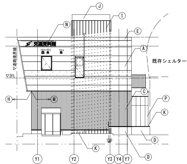
南側 立面図
