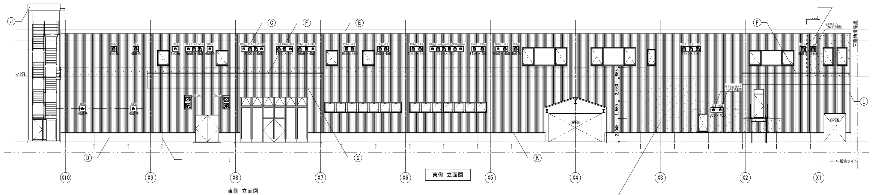
東側 立面図
