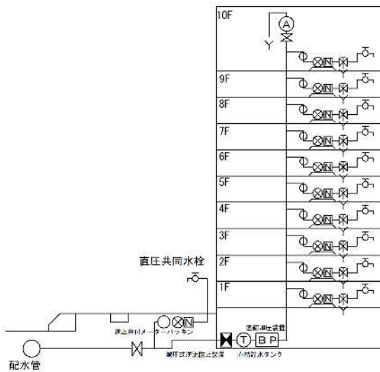
直結加圧 (増圧) 式 図 5-3
