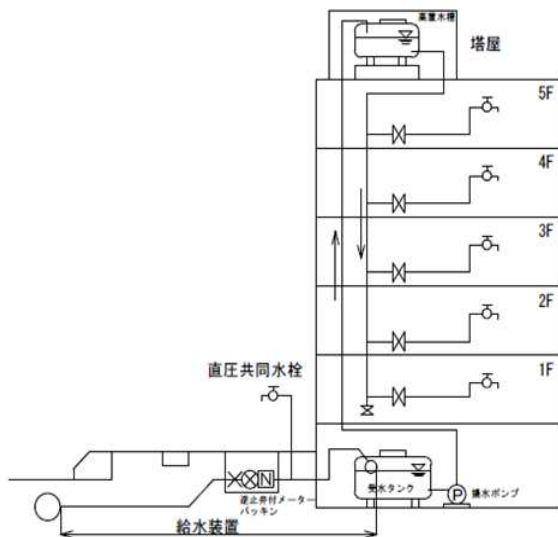
受水槽式 図 5-5
