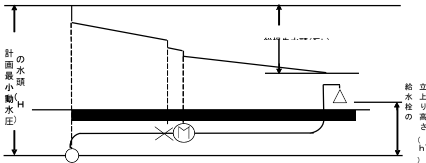
(h' + \sum h ) < H 水頭変化曲線図
