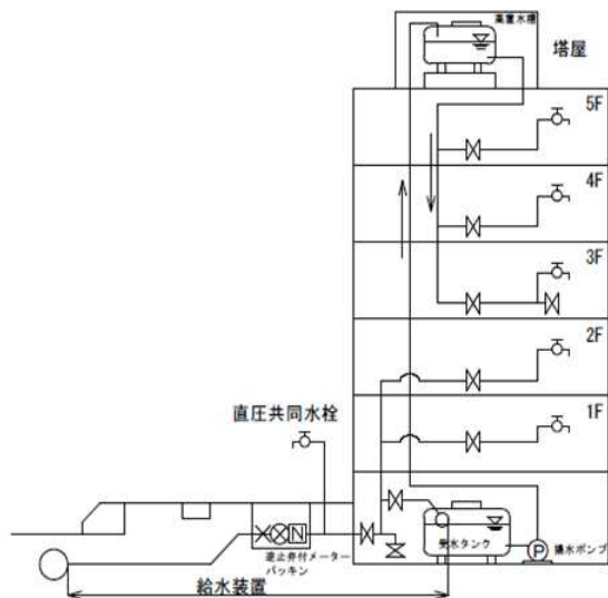
直結直圧・受水槽併用式 図 5-6
