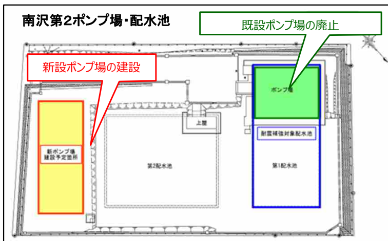
南沢第2ポンプ場・配水池 配置図 ※第2配水池は耐震性能あり (R1診断)
