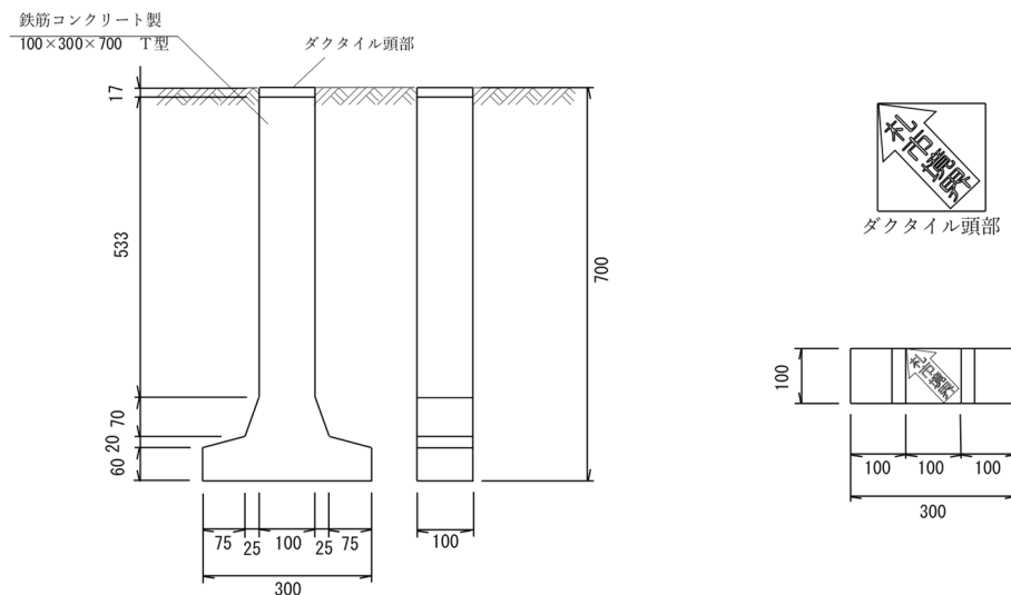
【側面図】
