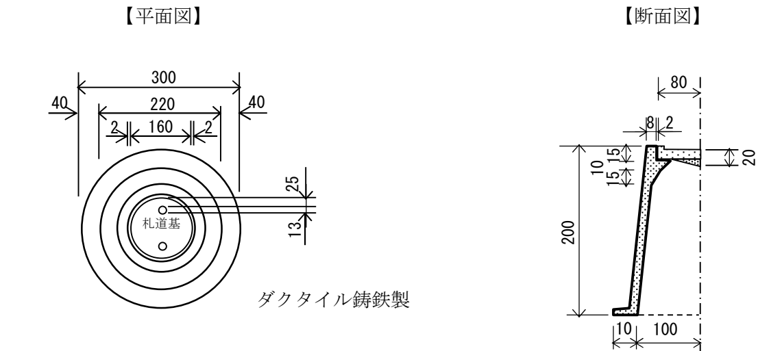
舗装路面用蓋 詳細図
