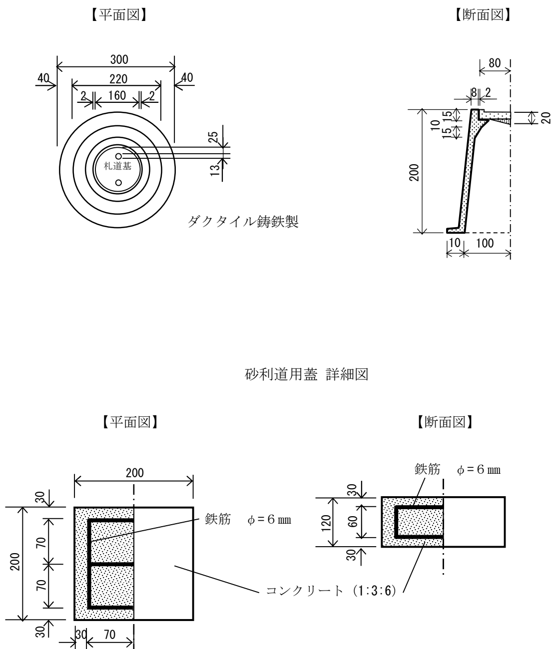
舗装路面用蓋 詳細図
