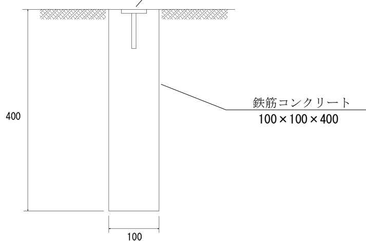
【側面図】
